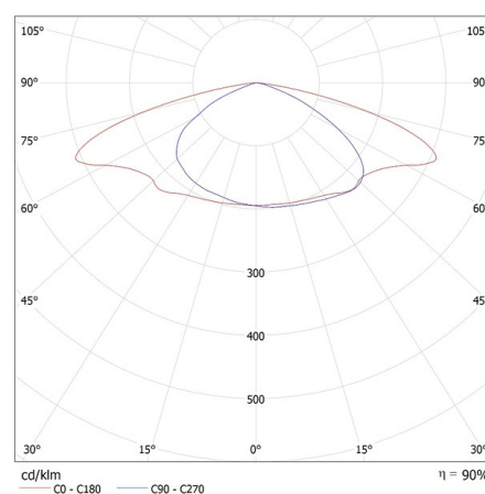
KANLUX S.A. (kat 39290) PRO-S S 15W-ZH NW / Krzywa rozsyłu światła (biegunowo)
